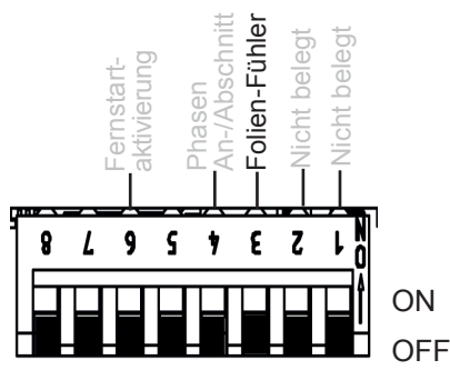
Abb. 12: Folienfühler
