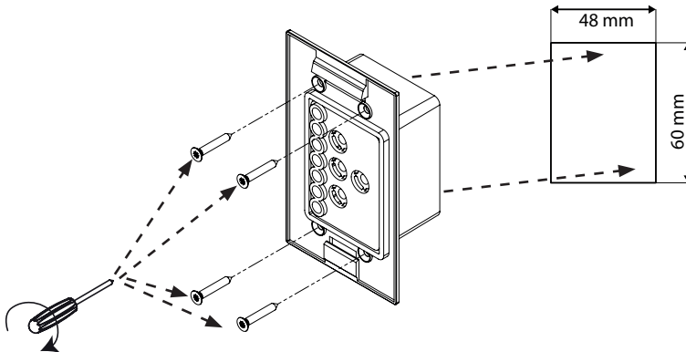
Abb.3 Montage Bedienteil
