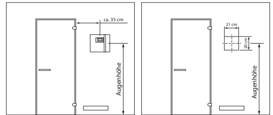
Wandausschnitt bei Montage in der Wand
