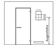
Wandausschnitt bei Montage in der Wand
