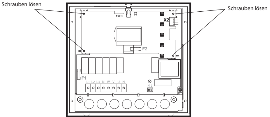
Display-Platine
