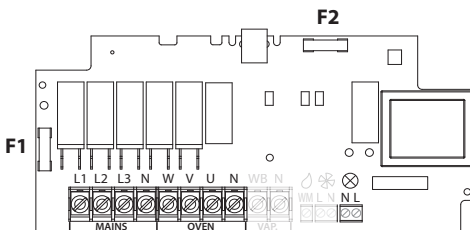
Hauptrelais-Platine
