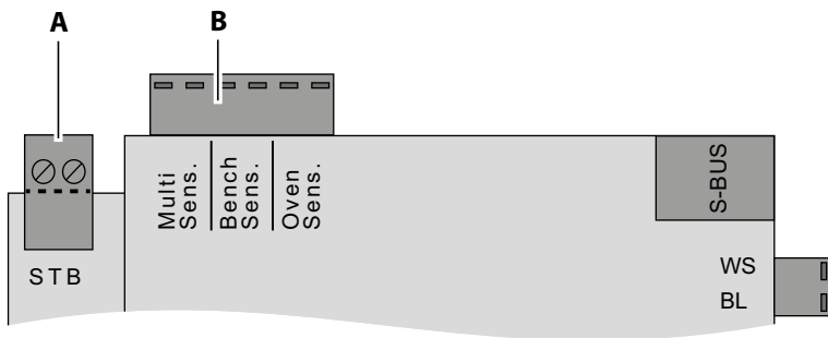
A Klemmenstecker STB
