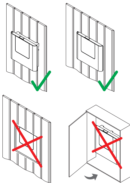
Richtige und falsche Montage des Steuergeräts
